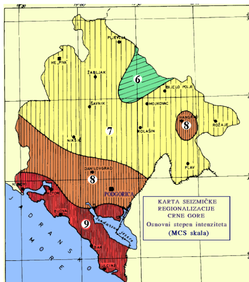
Slika 2 - Seizmička rejonizacija Crne Gore (V. Radulović, B. Glavatović, M. Arsović i V. Mihailov, 1982)
